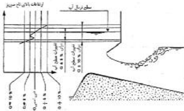
شکل ۲. پروفیل طولی جریان در یک دریچه از مدول تیغه‌ای
