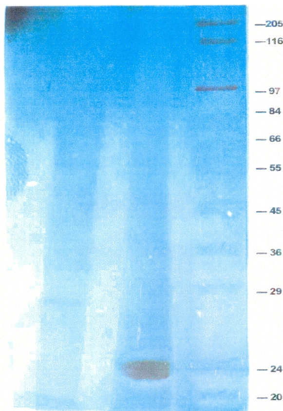
شکل ۵. نقش الکتروفورزی پروتئین جدایه مورد بررسی ALMV در ژل پلی اکریل آمیدی حاوی به ترتیب ستون اول مربوط به پروتئین‌های استاندارد، ستون دوم مربوط به آموده خالص شده ویروس و ستون سوم مربوط به آموده گیاه سالم
