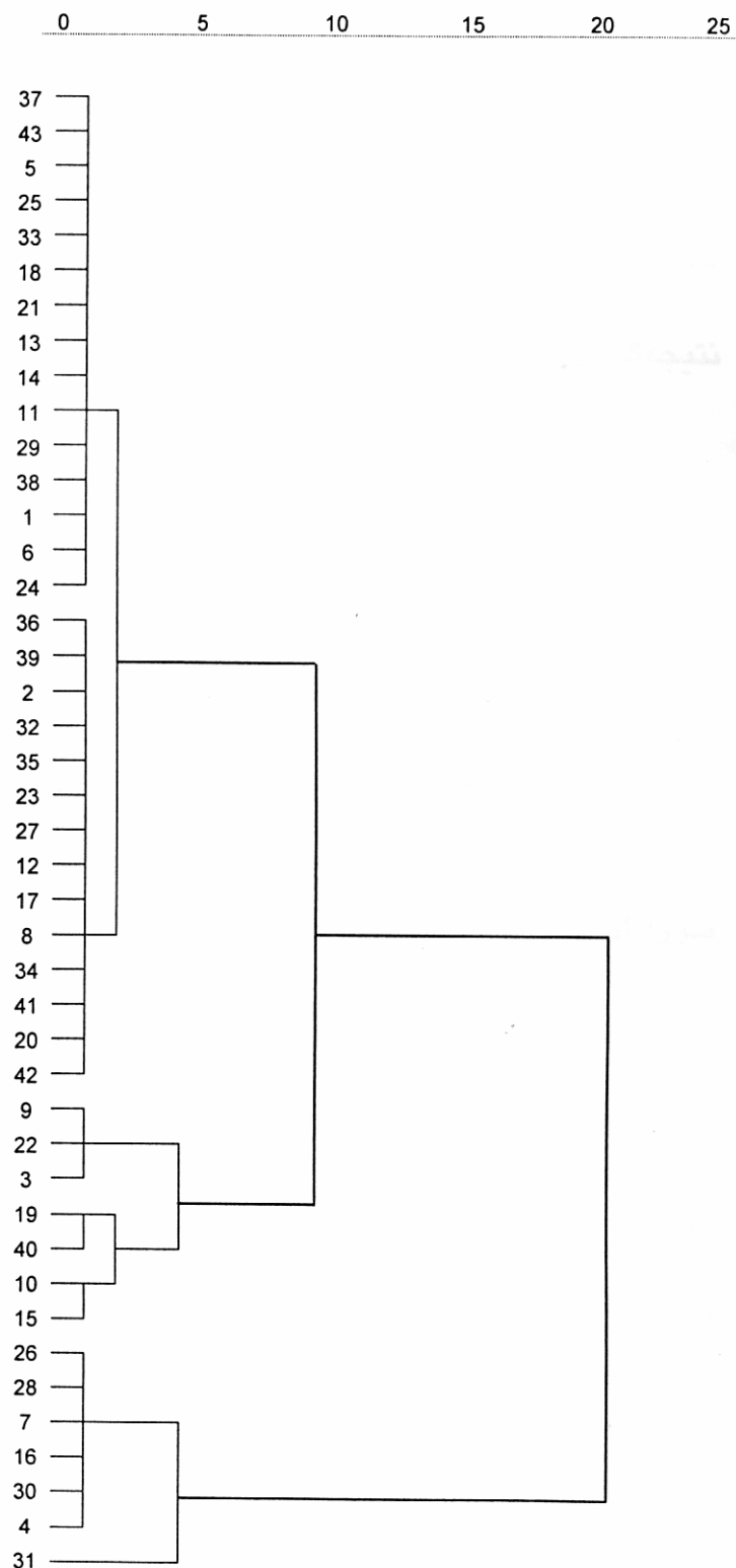
شکل ۱. دندروگرام حاصل از تجزیه کلاستر ۴۳ رقم گلایی به روش UPGMA در ارزیابی مزرعه‌ای با سیستم استاندارد USDA
