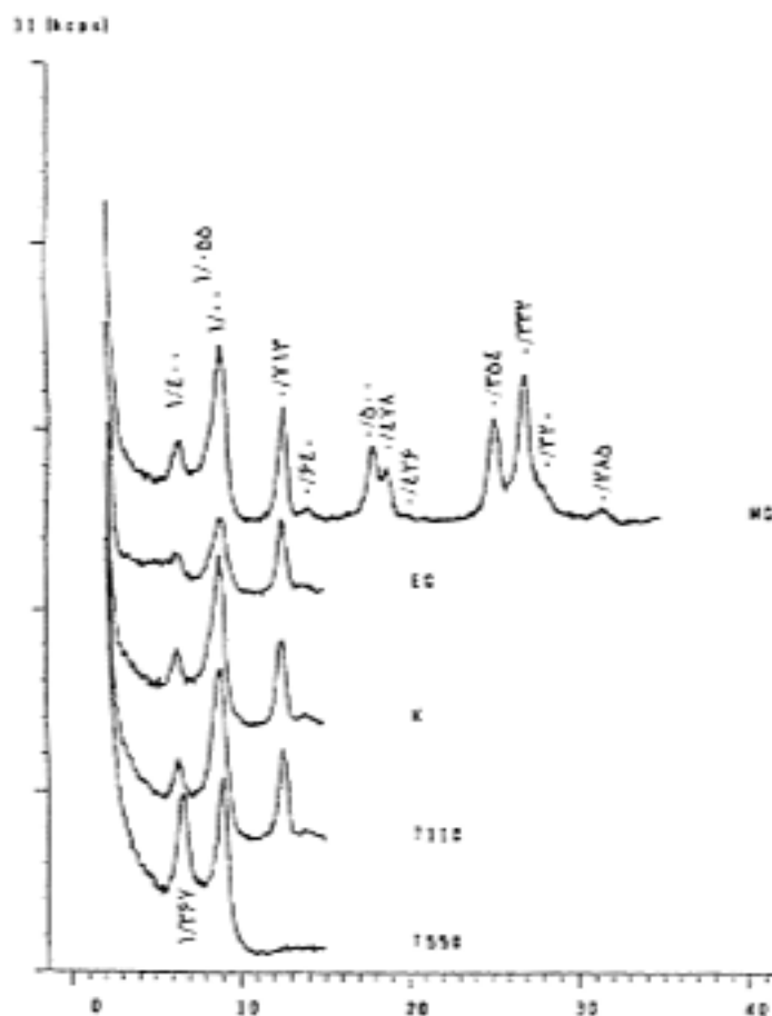
شکل ۳. پراش نگاشت‌های پرتو X ذرات رس درشت افق Byk-185 نیم‌رخ اول مخروط افکنه پایکوهی (A1)
