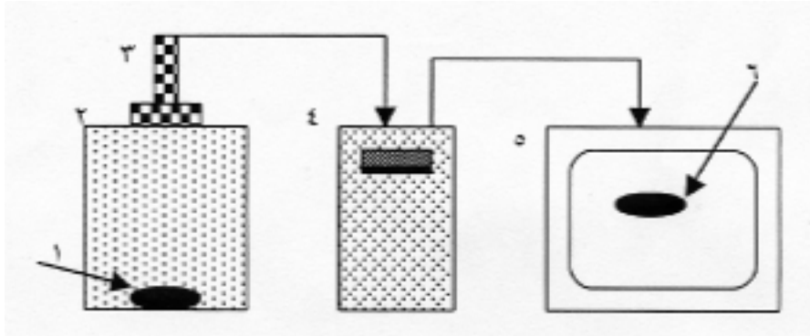
شکل ۱. طرح‌واره سیستم بینایی ماشین شامل دانه (۱)، جعبه نور (۲)، دوربین (۳)، رایانه (۴)، صفحه نمایش (۵)، و تصویر دانه (۶)
