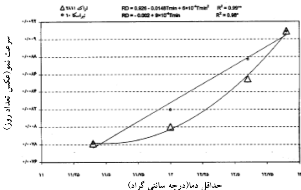
شکل ۵. ارتباط سرعت نمو با دمای حداقل در دوره کاشت تا رسیدگی فیزیولوژیک در ارقام اراک ۲۸۱۱ و نبراسکا ۱۰.
