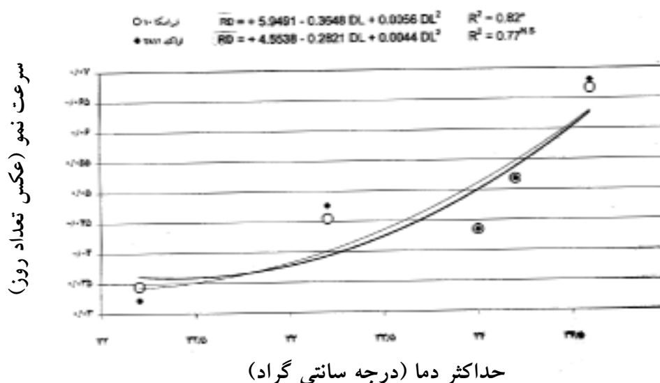
شکل ۱۲. ارتباط سرعت نمو با حداکثر دما در دوره رؤیت طبق تا شروع گلدهی در اراک ۲۸۱۱ و نبراسکا ۱۰.
