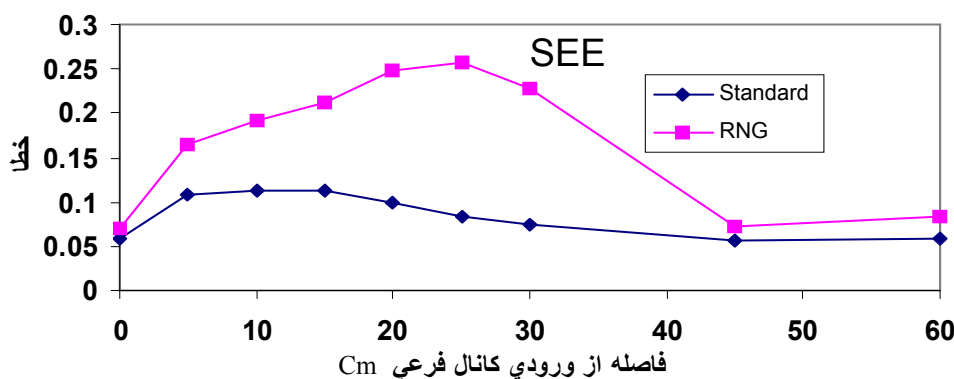
شکل ۹. خطای SEE در محاسبه سرعت در مقاطع مختلف کانال فرعی و برای عمق ۲۰ سانتی متر
