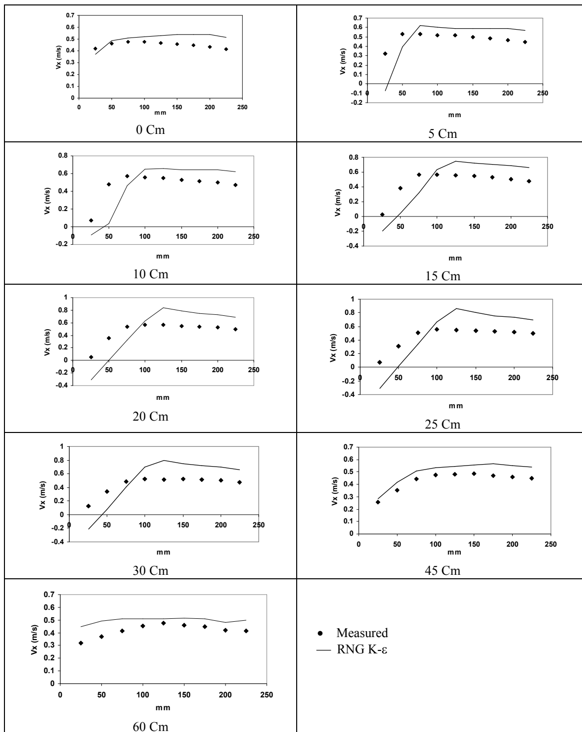
شکل ۸. مقایسه سرعت محاسبه شده در جهت جریان از مدل RNG K- \epsilon با مقادیر اندازه‌گیری شده در کانال فرعی و در مقاطع مختلف از ورودی برای عمق ۲۰ سانتی‌متر
