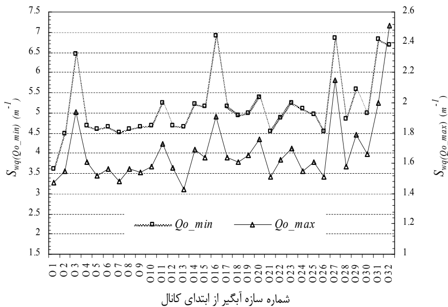
شکل ۶. مقادیر شاخص‌های حساسیت تغییرات نسبی بده به میزان بازشدگی سازه‌های آبگیر کانال وادودارا در بده‌های بهره‌برداری مورد مطالعه
