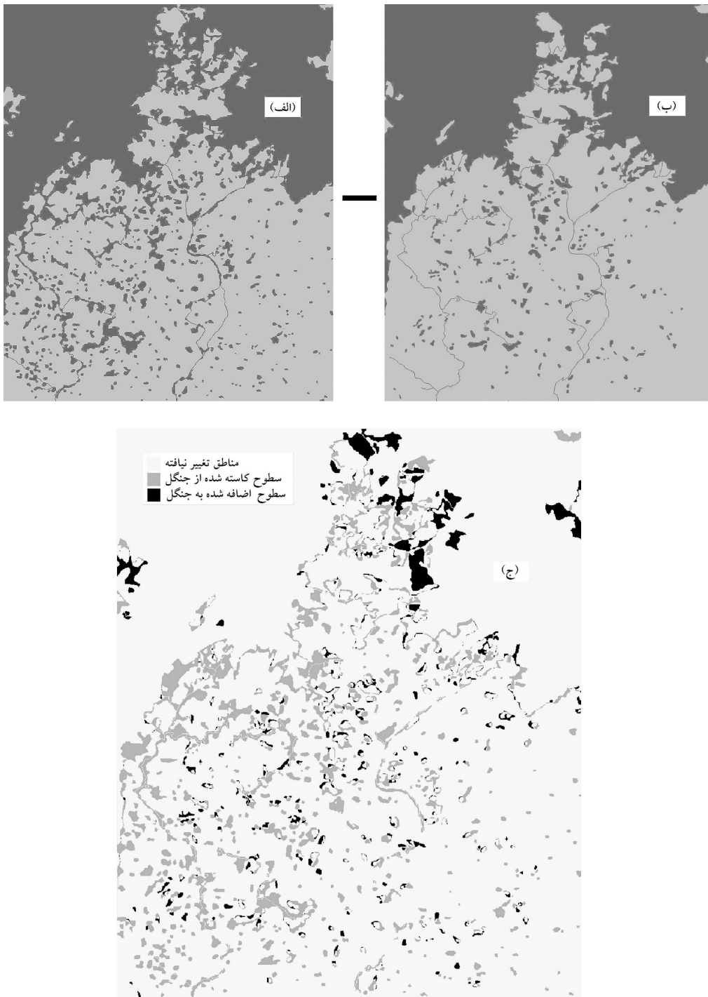
شکل ۳. نحوه تهیه نقشه تغییرات، نقشه جنگل حاصل از تفسیر تصویر ماهواره‌ای سال ۱۳۸۰ (الف)، نقشه جنگل مربوط به سال ۱۳۷۳ (ب) استخراج شده از نقشه توپوگرافی (ب)، نقشه تغییرات سطح جنگل که از تفریق دو نقشه مذکور به دست آمده است (ج).
