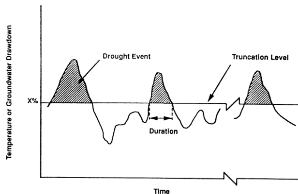
شکل ۲. نمایش مفهوم خشکسالی در روش Chang برای معرف‌های دما و آب زیرزمینی (۷)
