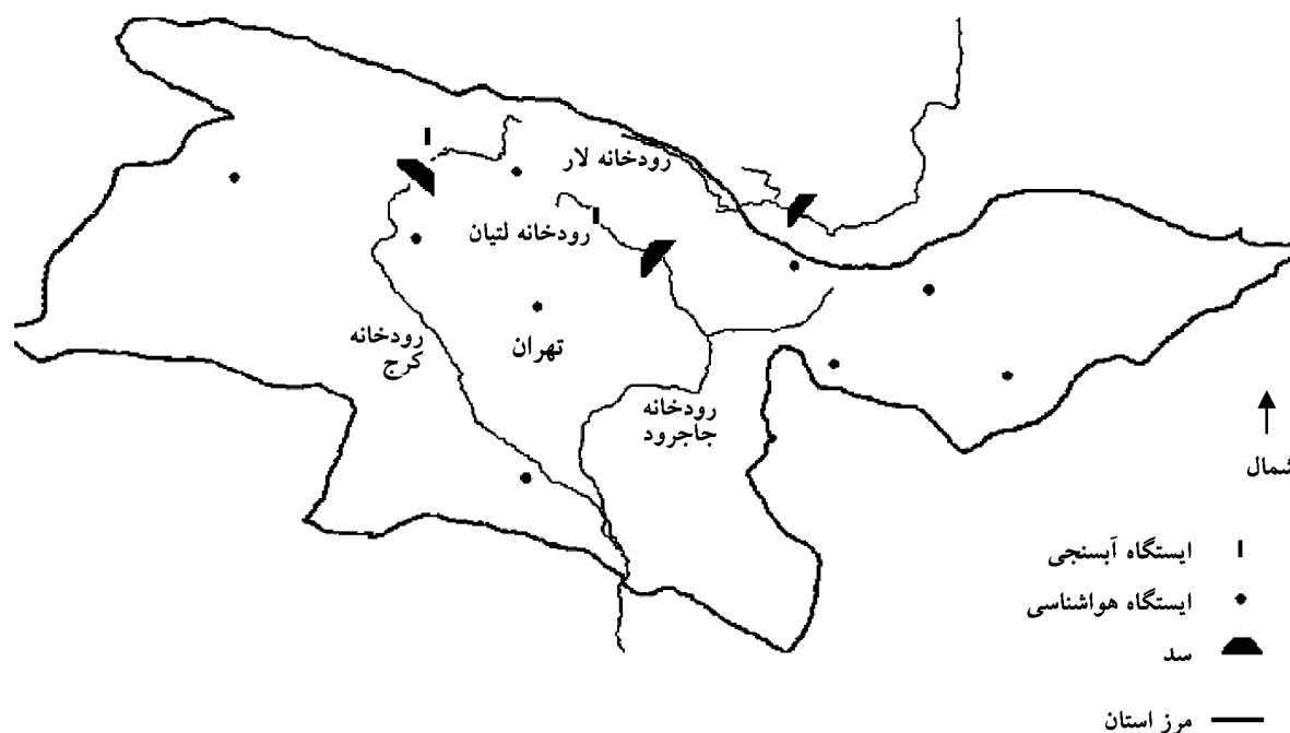
شکل ۱. موقعیت استان تهران و سامانه اصلی منابع آب آن
