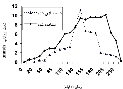
شکل ۴. منحنی واسنجی هیدروگراف برای مدل EUROSEM قبل (الف) و بعد (ب) از واسنجی به وسیله رخداد ۲۶ فروردین ۱۳۸۲ در حوضه سوليجان
