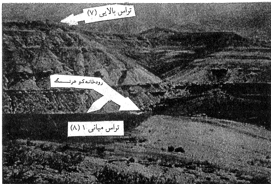
شکل ۳. نمایشی از وضع زمین‌نمای تراس‌ها در اطراف رود کوه‌رنسگ (ناحیه اقلیمی چلگرد)
