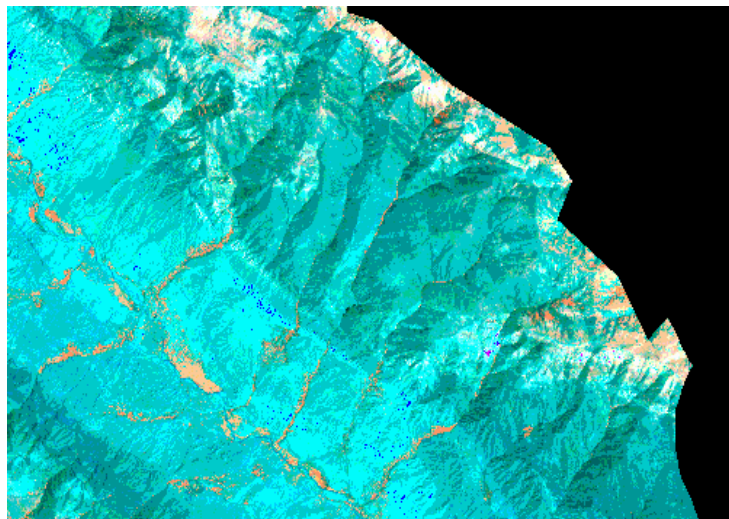
شکل ۲. تصویر تهیه شده براساس ترکیب سه باند PCA1, PCA3 , \lambda_3
