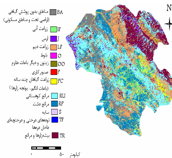
شکل ۶. نقشه تهیه شده براساس ترکیب ۱.۵، ۱.۴، ۱.۳ به روش حداکثر همانندی
