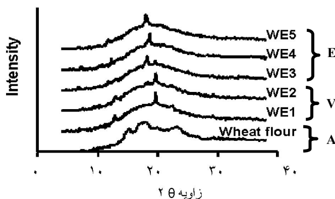
شکل ۱۰. الگوی X-ray انکساری نمونه‌های اکسترود شده نشاسته گندم با SME های متفاوت WE1 (تا WE5) در مقایسه با آرد گندم
