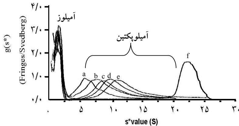
شکل ۱۳. نمودار ته‌نشین شدن آمیلوز و آمیلوپکتین اکستروده شده نشاسته گندم با SMEهای متفاوت. حروف e تا a به ترتیب مربوط به نمونه‌های اکستروده شده WE1 تا WE5 می‌باشد و نمونه f شاهد (آرد گندم) است
