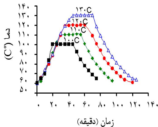
شکل ۱. نمودار دما - زمان نمونه‌های نشاسته گندم اتوکلاو شده در دماهای ۱۰۰-۱۳۰ °C و فشار ۱۵psi
