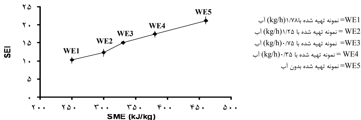
شکل ۷. تغییرات انبساط حجمی نمونه‌های اکسترودر شده نشاسته گندم در SMEهای مختلف
