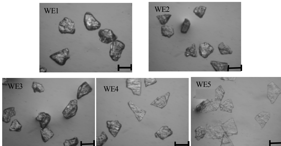
شکل ۹. میکروگراف نمونه‌های اکسترود شده نشاسته گندم با SME های متفاوت (خط زیر هر شکل ۱۰۰ μm است). WE1 = نمونه تهیه شده با ۱/۷۸ (kg/h) آب، WE2 = نمونه تهیه شده با ۱/۲۵ (kg/h) آب، WE3 = نمونه تهیه شده با ۰/۷۵ (kg/h) آب، WE4 = نمونه تهیه شده با ۰/۳۵ (kg/h) آب و WE5 = نمونه تهیه شده بدون آب.
