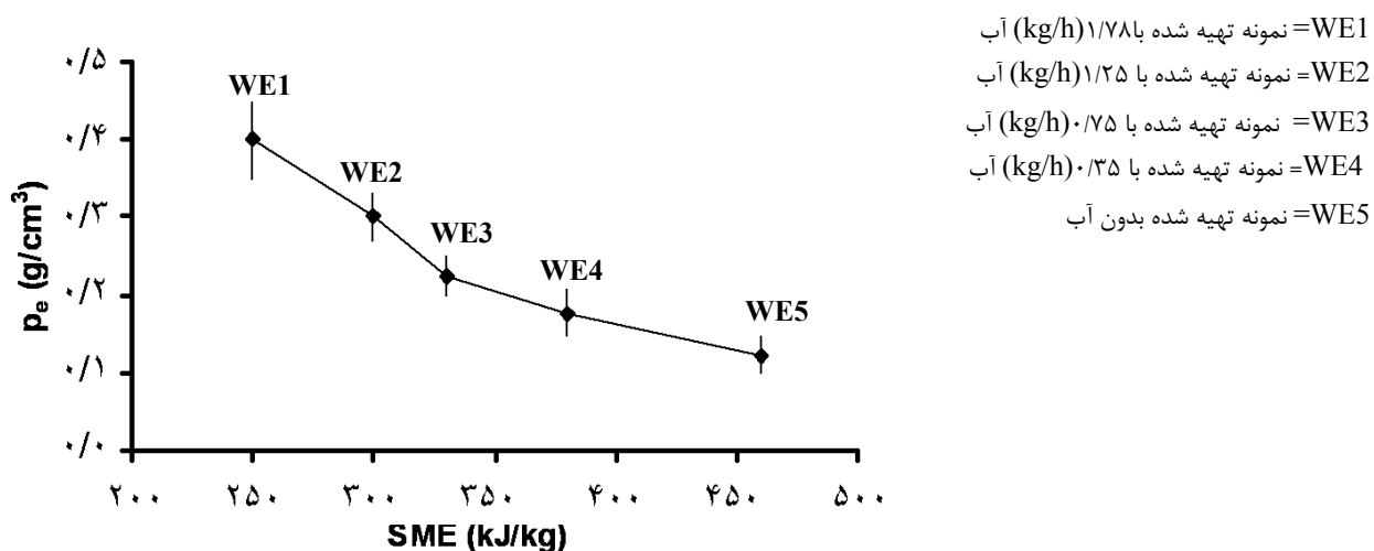
شکل ۸. تغییرات دانسیته نمونه‌های اکسترودر شده نشاسته گندم در SMEهای مختلف
