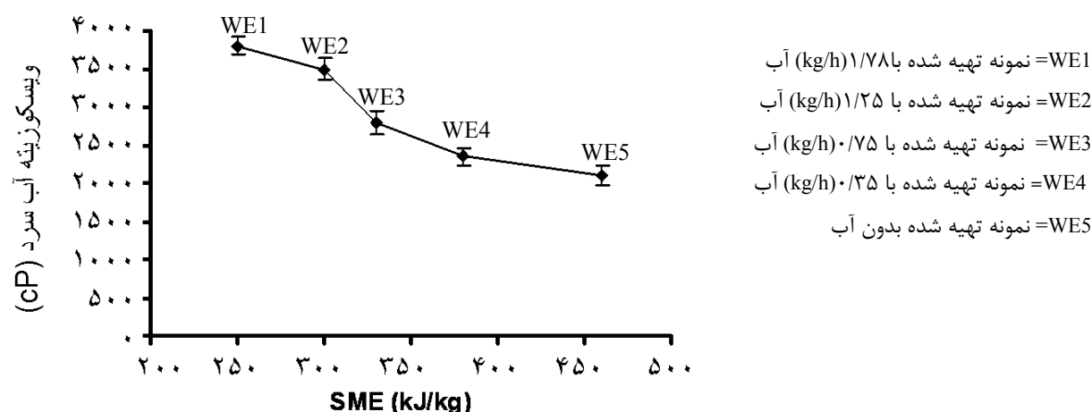
شکل ۱۲. نمودار ویسکوزیته نهایی نمونه‌های اکستروژ شده نشاسته گندم (پس از سرد شدن خمیر در دستگاه RVA تا دمای 25^{\circ}\text{C} ) با SMEهای متفاوت
