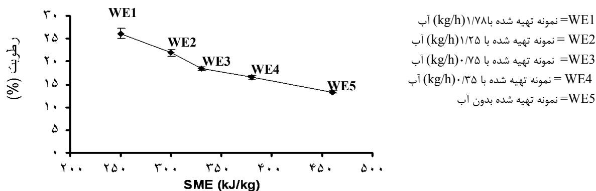
شکل ۶. تغییرات SME با میزان آب مصرفی جهت تهیه نمونه‌های نشاسته گندم در اکسترودر
