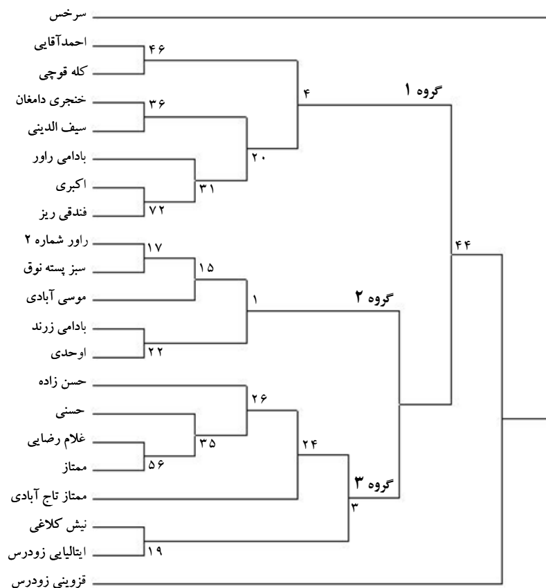
شکل ۳. گروه‌بندی ژنوتیپ‌های پسته ایرانی بر اساس الگوهای باندی SSR. با استفاده از ضریب تشابه نی (۱۹۸۳) و روش UPGMA. ضرایب هر Internal node مربوط به آزمون Bootstrap است.
