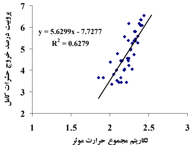
شکل ۶. رابطه خطی بین پرویت درصد ظهور حشرات کامل پروانه چوبخوار پسته و لگاریتم مجموع حرارت مؤثر برای ظهور حشرات کامل بر اساس آستانه حداقل حرارتی ۱۱ درجه سانتی گراد در شرایط صحرائی
