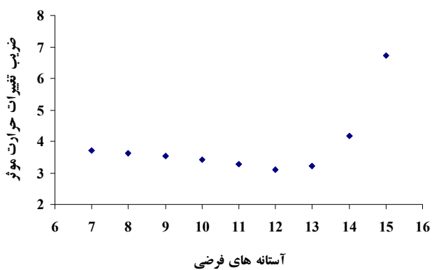
شکل ۳. ضریب تغییرات حرارت مؤثر با توجه به آستانه‌های فرضی مختلف برای ۵۰٪ تشکیل پيله شفیرگی تا ۵۰٪ ظهور حشرات کامل در مطالعات صحرائی
