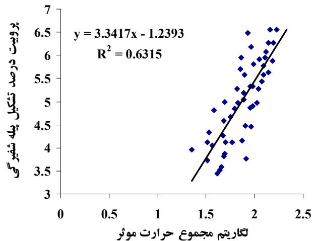
شکل ۴. رابطه خطی بین پرویت درصد تشکیل پیله شفیرگی پروانه چوبخوار پسته و لگاریتم مجموع حرارت مؤثر برای تشکیل پیله شفیرگی بر اساس آستانه حداقل حرارتی ۱۰ درجه سانتی گراد در شرایط صحرائی
