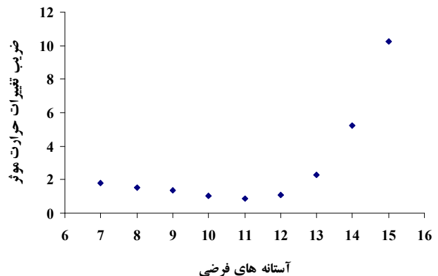
شکل ۲. ضریب تغییرات حرارت مؤثر با توجه به آستانه‌های فرضی مختلف برای لارو تا ۵۰٪ ظهور حشرات کامل در مطالعات صحرائی
