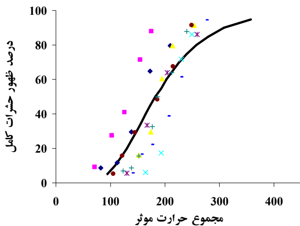
شکل ۷. مجموع حرارت مؤثر لازم برای درصدهای ظهور حشرات کامل پروانه چوبخوار پسته از لارو زمستان گذران بر اساس آستانه حداقل حرارتی ۱۱ درجه سانتی گراد در شرایط صحرائی
