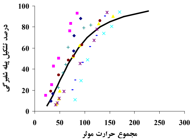
شکل ۵. مجموع حرارت مؤثر لازم برای درصدهای تشکیل پیله شفیرگی پروانه چوبخوار پسته از لارو زمستان گذران بر اساس آستانه حداقل حرارتی ۱۰ درجه سانتی گراد در شرایط صحرائی
