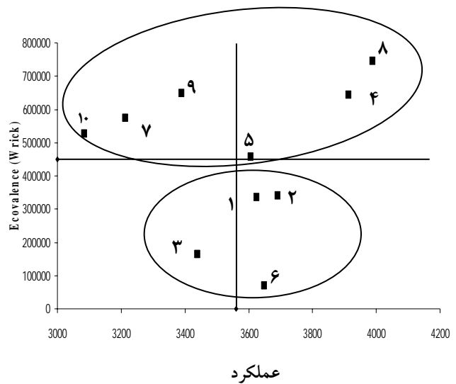
شکل ۱. بای پلات پراکنش ژنوتیپ‌ها از نظر دو پارامتر میانگین عملکرد وش و واریانس محیطی
