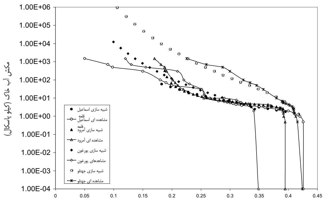
شکل ۲. مقادیر اندازه‌گیری و شبه‌سازی شده منحنی مشخصه آب خاک در بافت‌های شنی، لوم رسی شنی، شنی لومی و لوم رسی لایی (به ترتیب در سری‌های اسماعیل قلعه، امرود آغاچ، بورغون آباد و جهتلو)
