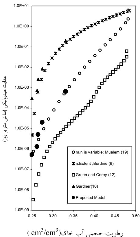
شکل ۱۰. هدایت هیدرولیکی در خاک مبارک آباد (بافت رسی)
