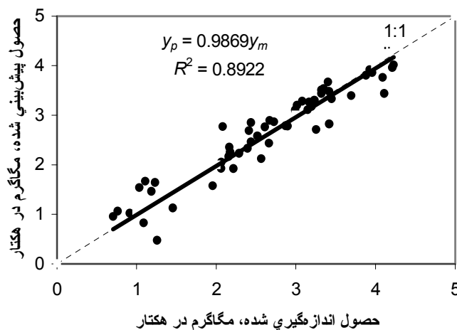
شکل ۴. مقادير اندازه گيري شده ( y_m ) و پيش بيني شده ( y_p ) عملکرد گندم در برابر آب آبياري و باران فصل رشد و نيتروژن اوليه و مصرفي
